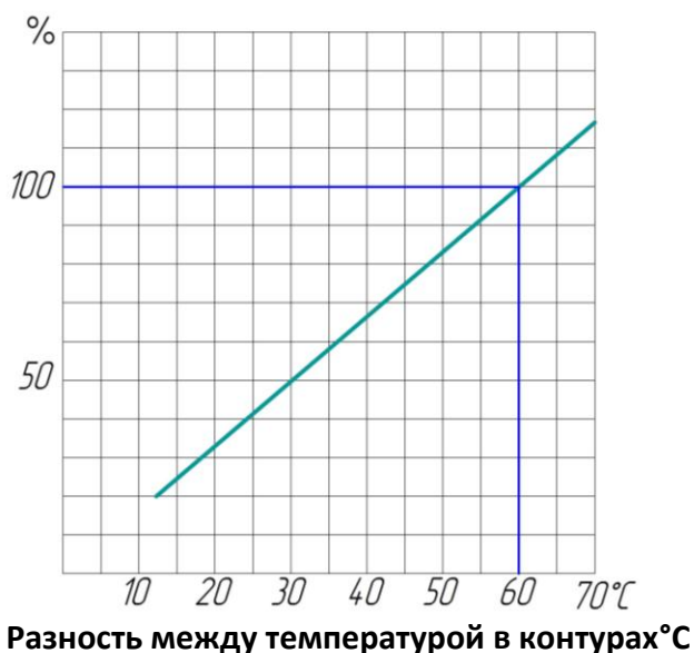
Диаграмма А (Номинальная тепловая мощность%)
